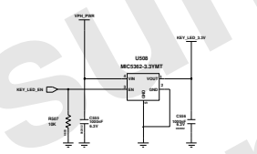
KEYLED LDO(150mA)
